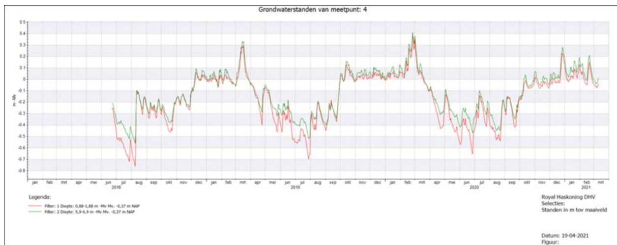
Afbeelding 7.3-1: Verdrogingsmeetpunt in het Natura 2000-gebied Van Oordt's Mersken, Koningsdiep. Bij dit meetpunt wordt op twee verschillende dieptes de grondwaterstand (stijghoogtes) gemeten.
