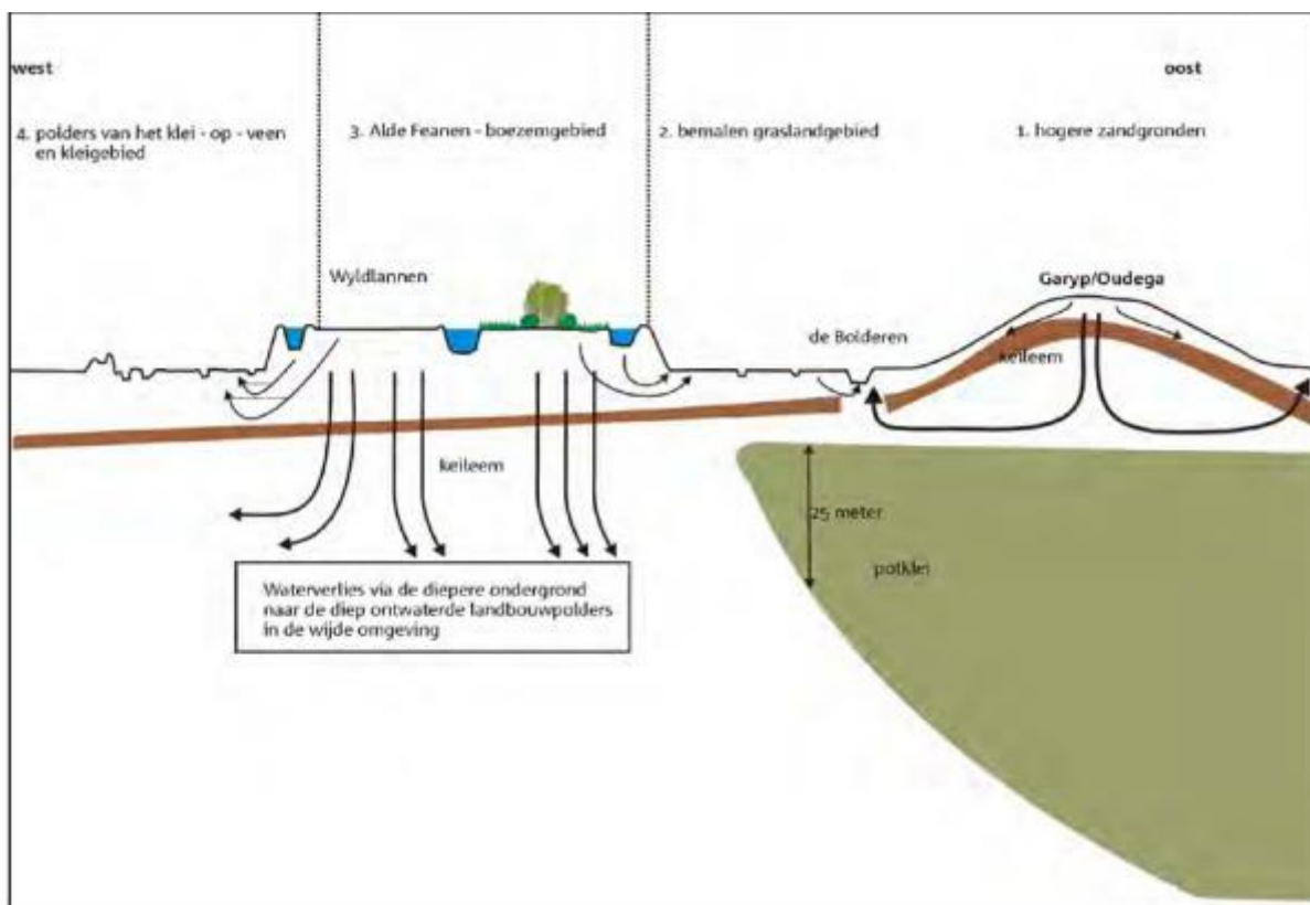
Figuur 1-1: Conceptuele illustratie van het hydrologische systeem.
